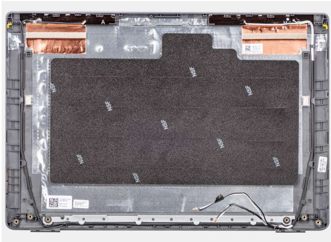
Ilustración 69. Instalación de la cubierta posterior de la pantalla
