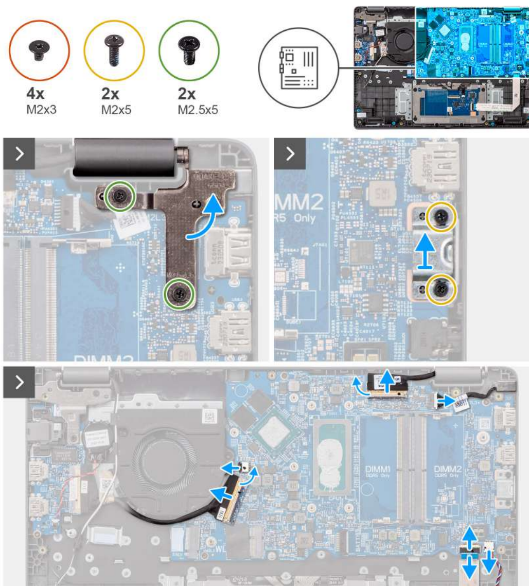
Ilustración 42. Extracción de la tarjeta madre
