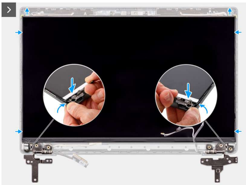
Ilustración 62. Instalación del panel de pantalla
