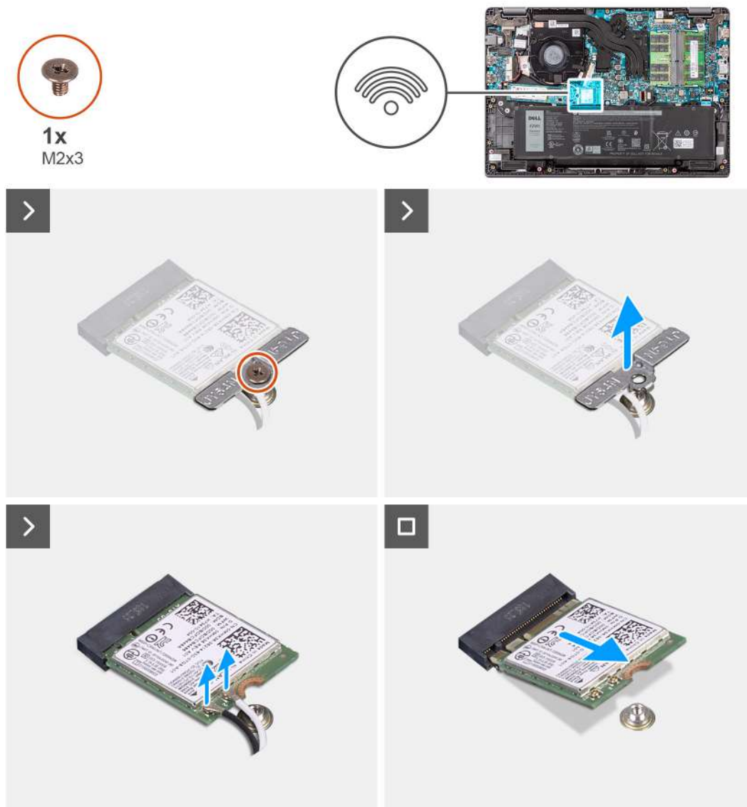
Ilustración 15. Extracción de la tarjeta inalámbrica
