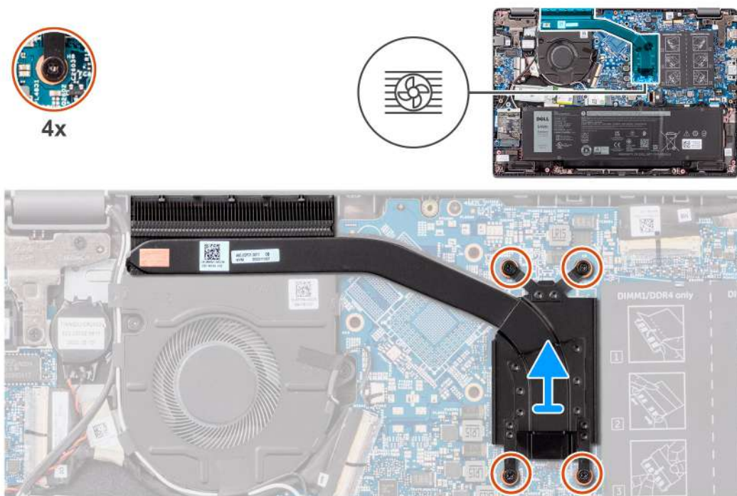
Ilustración 29. Extracción del disipador de calor para gráficos integrados
