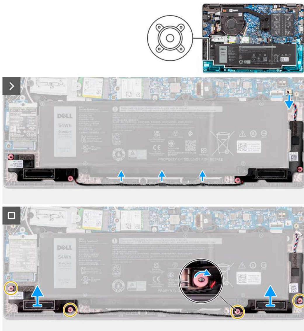
Ilustración 21. Extracción de los parlantes
