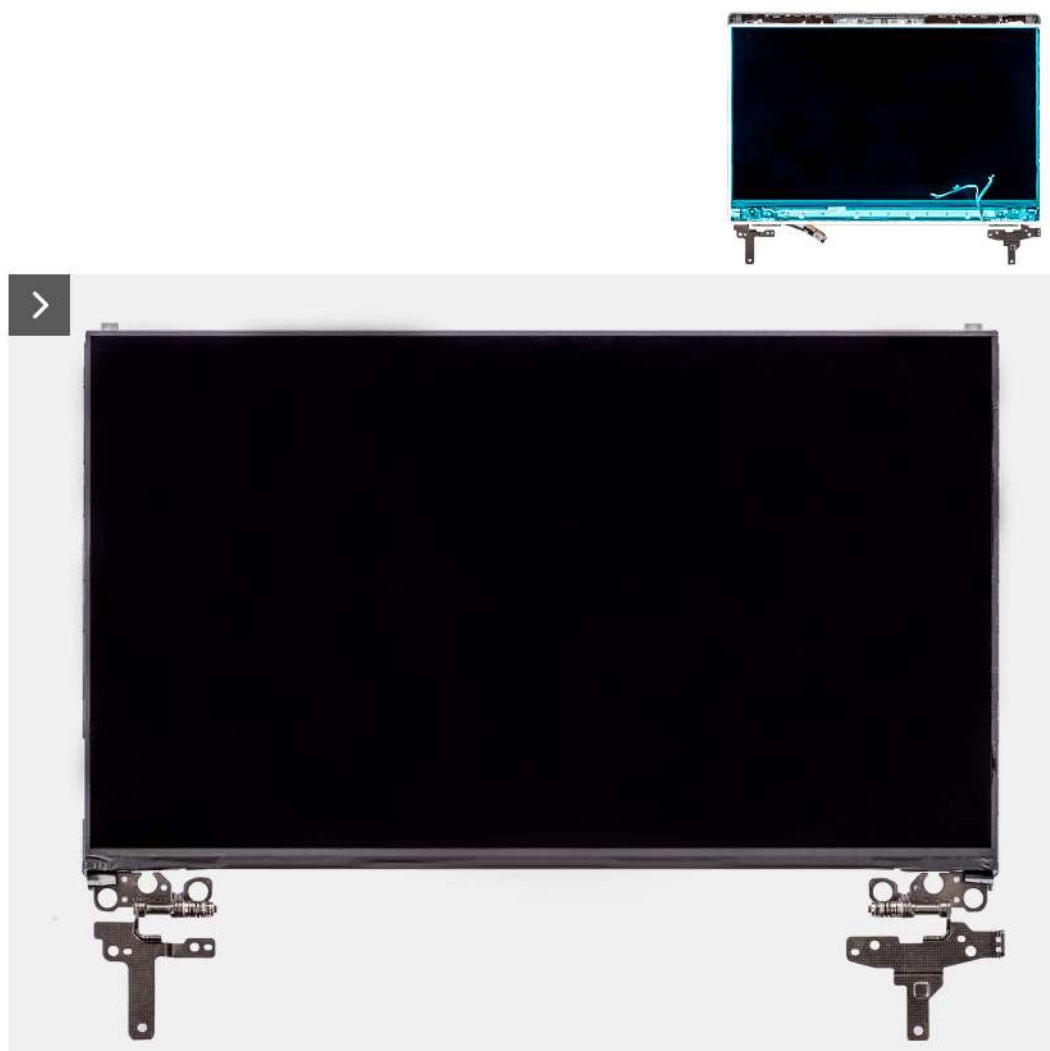
Ilustración 59. Instalación del panel de pantalla
