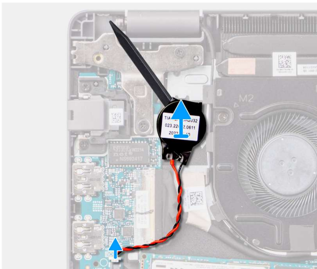
Ilustración 17. Extracción de la batería de tipo botón
