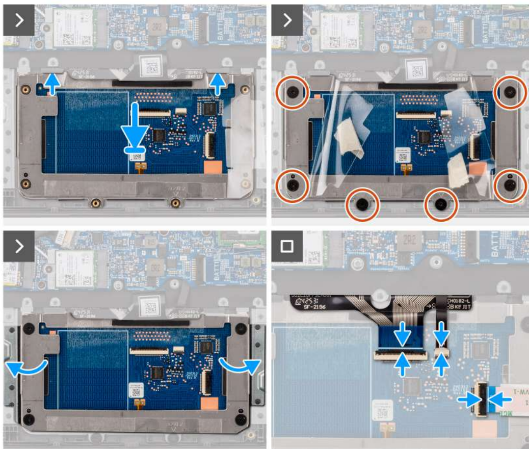
Ilustración 36. Instalación del panel táctil
