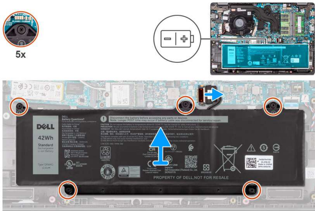
Ilustración 23. Extracción de la batería
