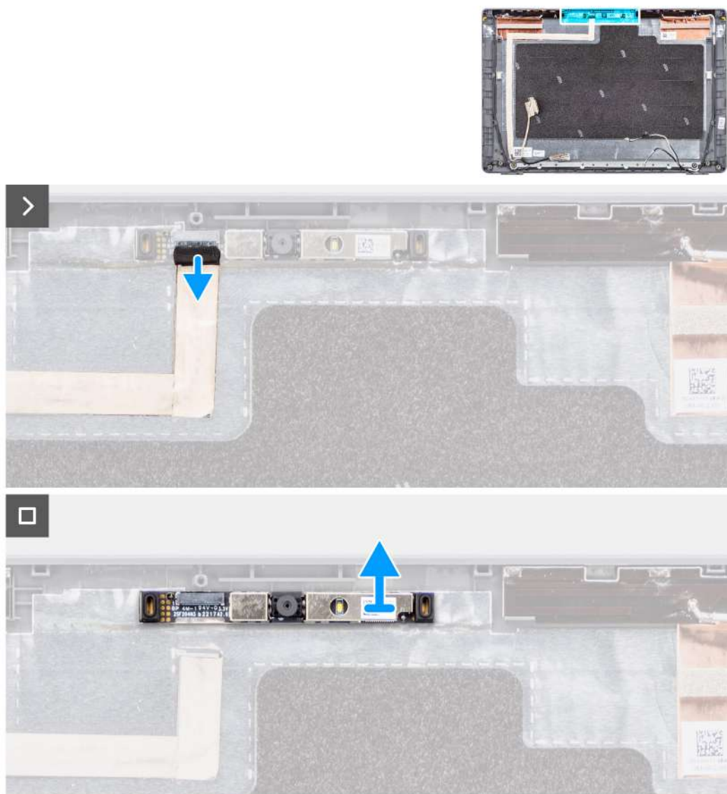
Ilustración 64. Extracción de la cámara
