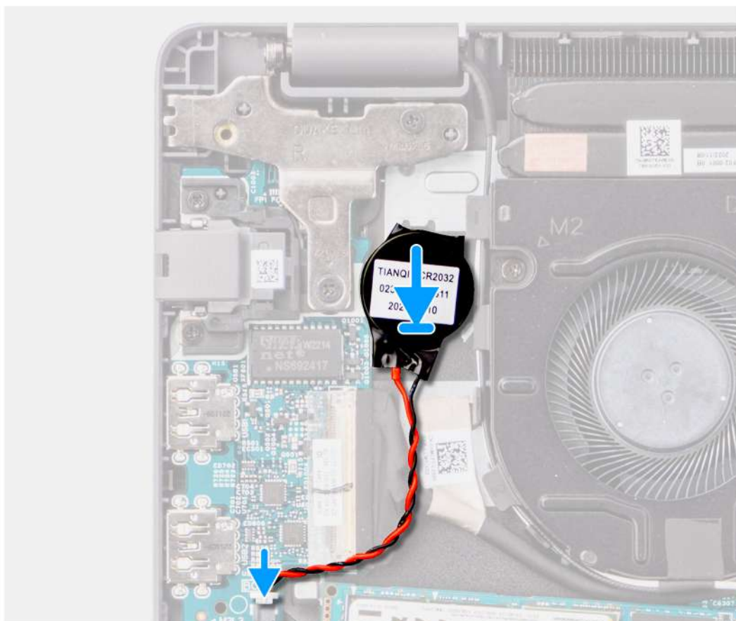
Ilustración 18. Instalación de la batería de tipo botón
