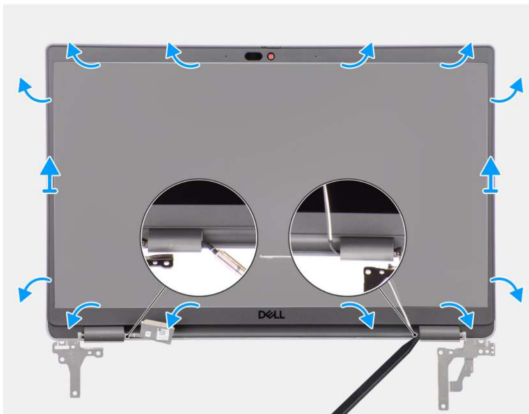
Ilustración 52. Extracción del bisel de la pantalla
