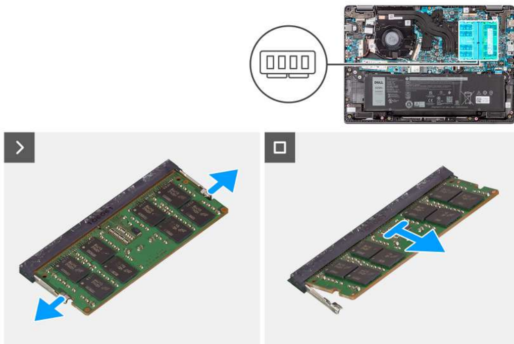
Ilustración 13. Extracción del módulo de memoria
