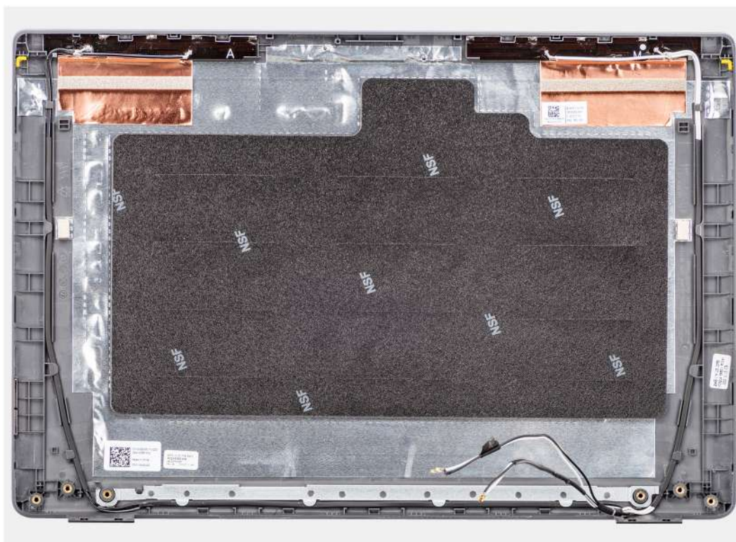
Ilustración 68. Extracción de la cubierta posterior de la pantalla
