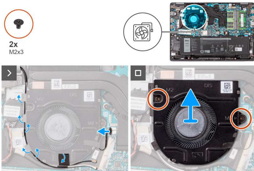
Ilustración 33. Extracción del ventilador
