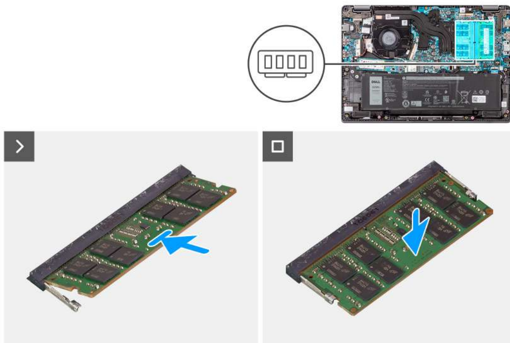
Ilustración 14. Instalación de los módulos de memoria
