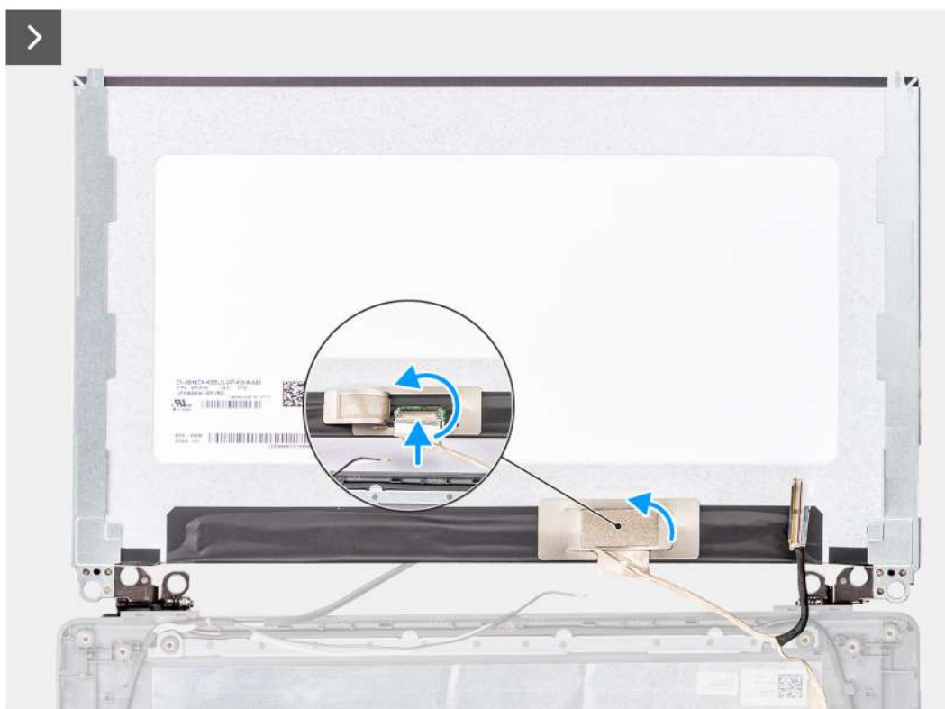
Ilustración 60. Instalación del panel de pantalla
