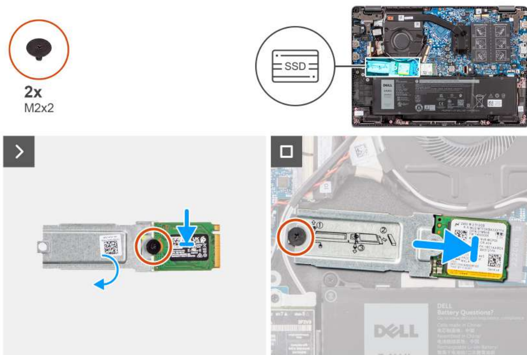
Ilustración 20. Instalación de la unidad de estado sólido M.2 2230
