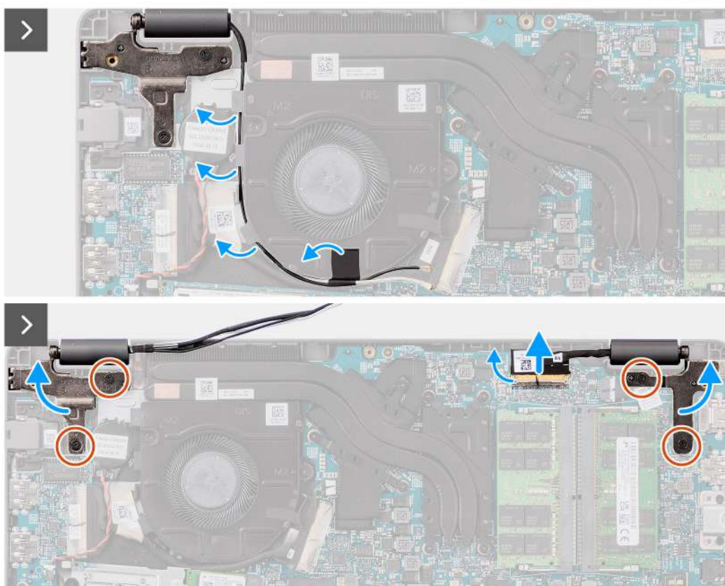
Ilustración 47. Extracción del ensamblaje de la pantalla
