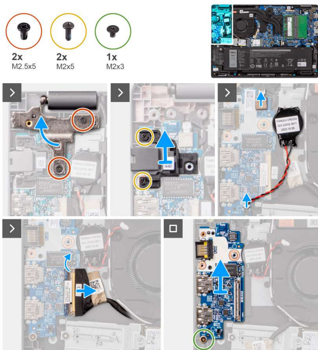
Ilustración 37. Extracción de la placa de I/O
