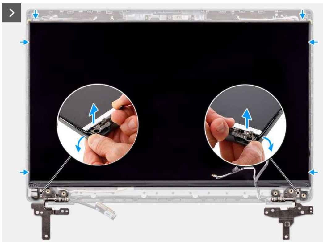
Ilustración 55. Extracción del panel de pantalla
