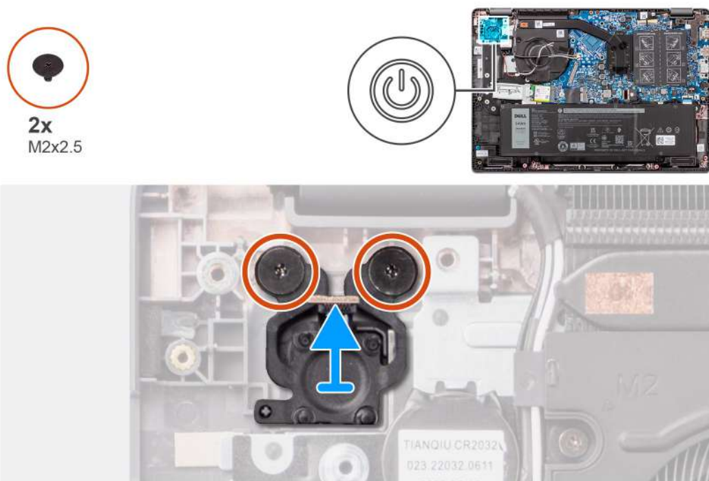
Ilustración 39. Extracción del botón de encendido
