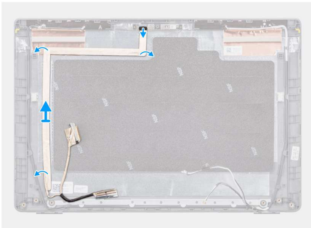
Ilustración 66. Extracción del cable de eDP
