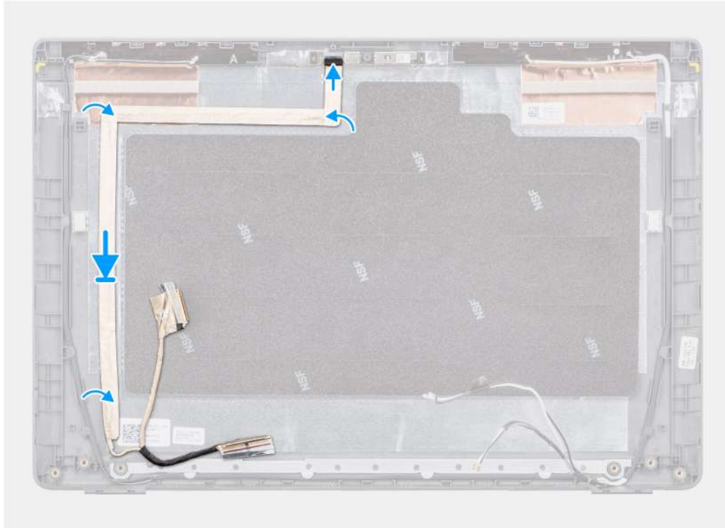
Ilustración 67. Instalación del cable eDP
