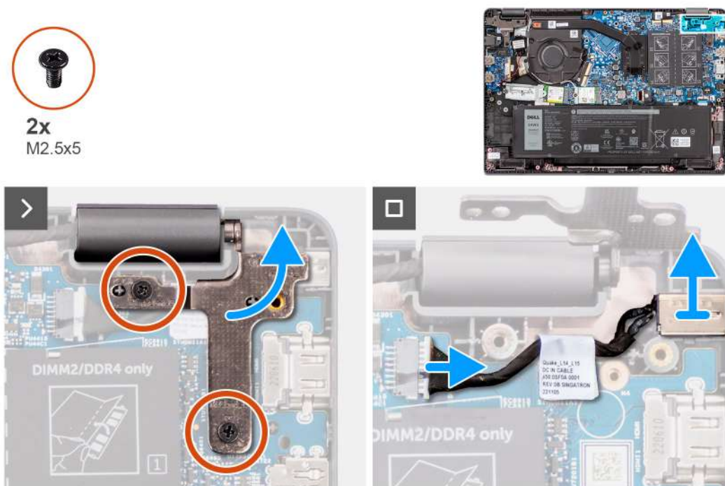
Ilustración 27. Extracción del puerto del adaptador de alimentación
