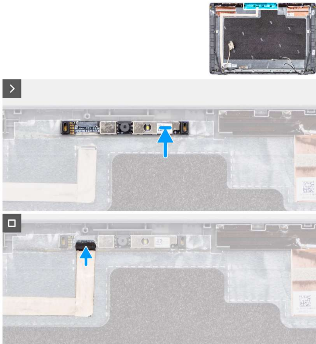
Ilustración 65. Instalación de la cámara
