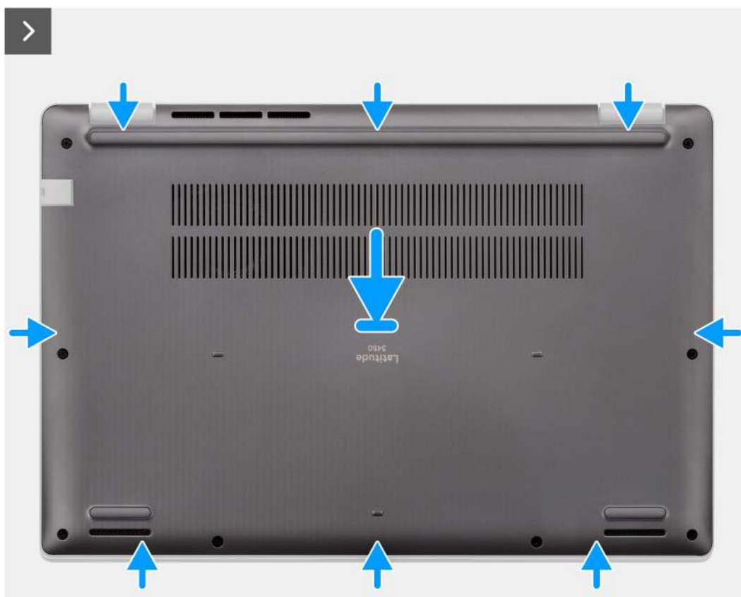
Ilustración 11. Instalación de la cubierta de la base
