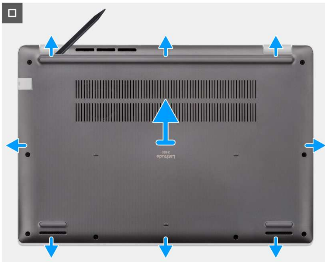
Ilustración 10. Extracción de la cubierta de la base
