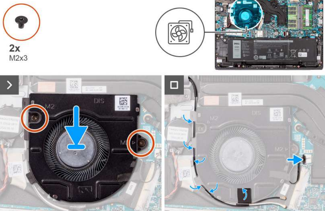
Ilustración 34. Instalación del ventilador
