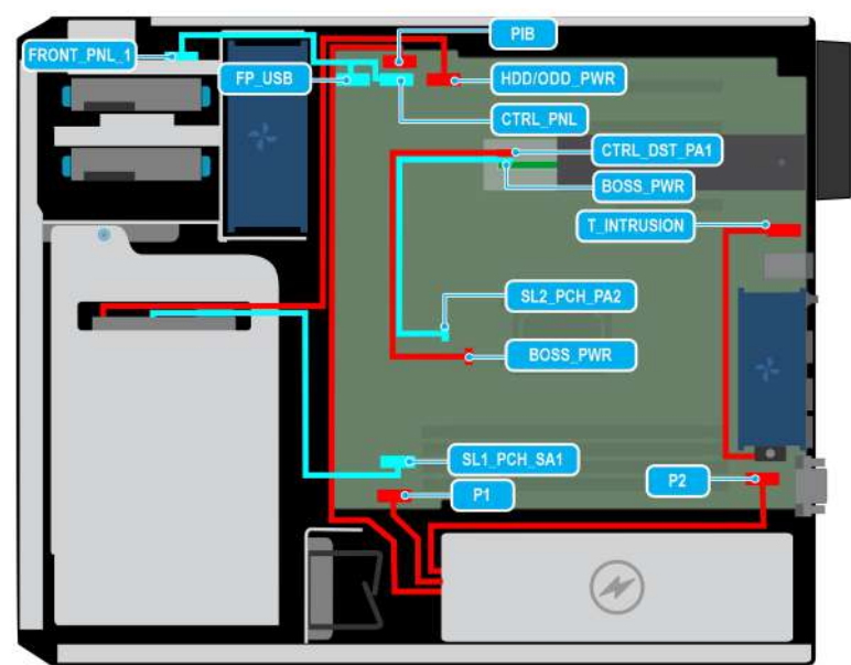
Ilustración 30. Colocación de cables: 3 SATA con chip de 3,5 pulgadas
