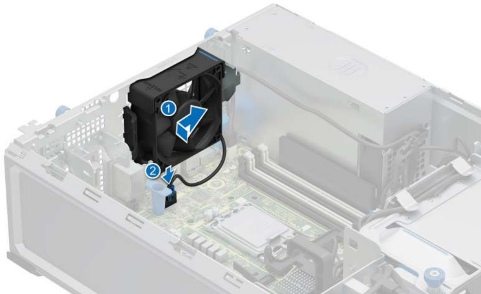
Ilustración 28. Instalación del ventilador de enfriamiento
