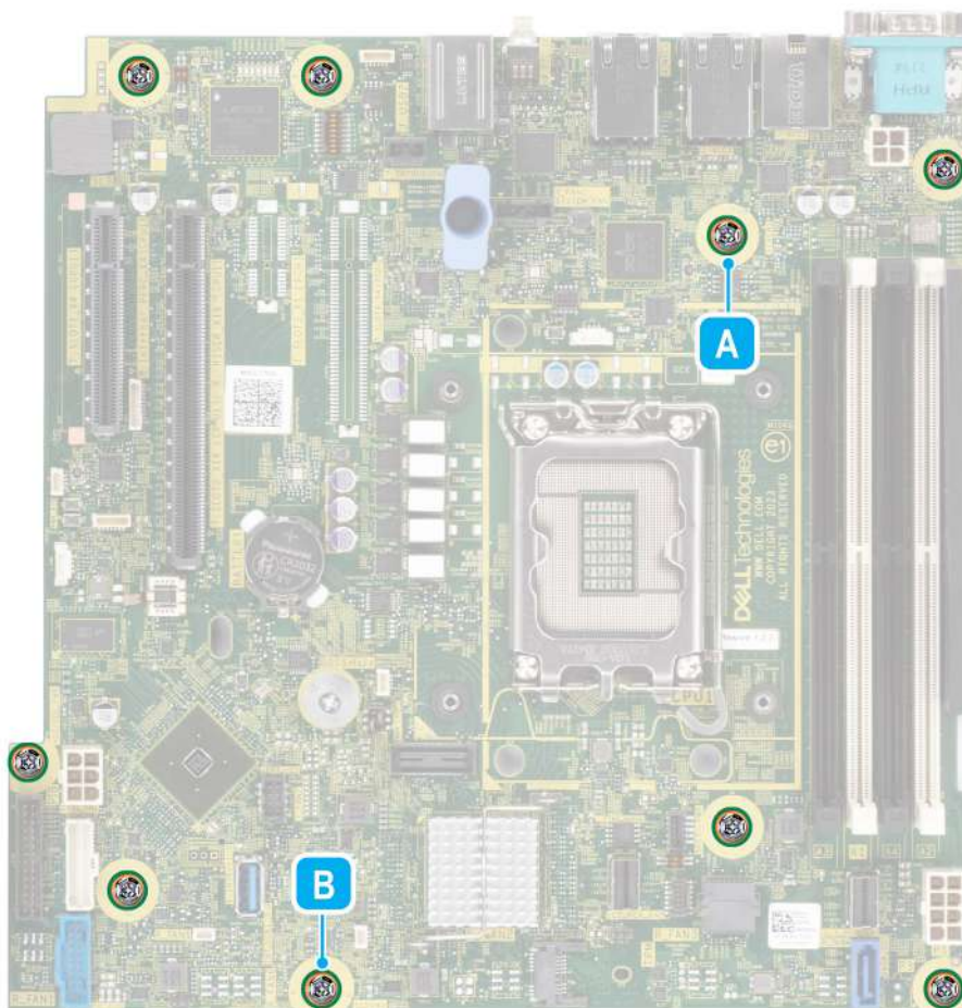
Ilustración 64. Ubicación del tornillo de la tarjeta madre
