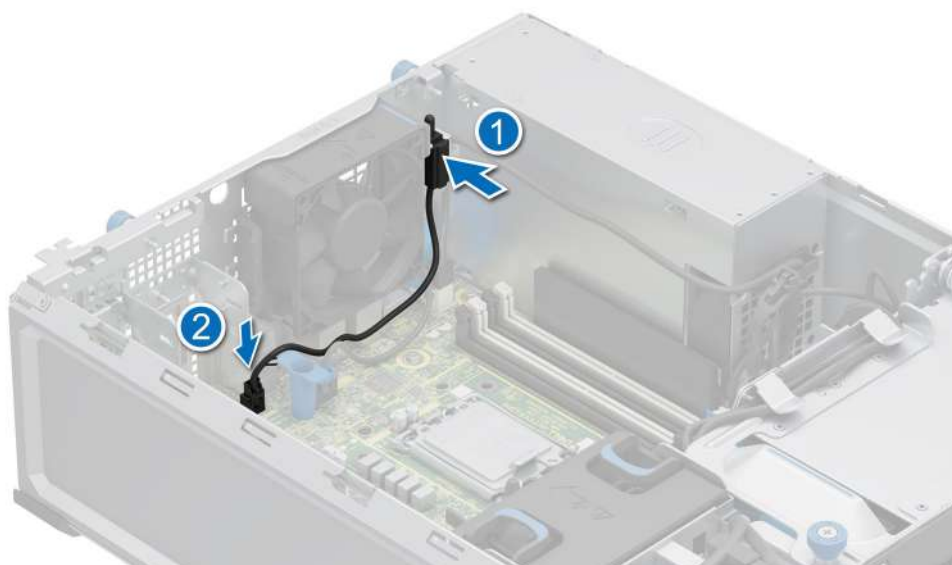
Ilustración 17. Instalación del módulo del switch de intrusión
