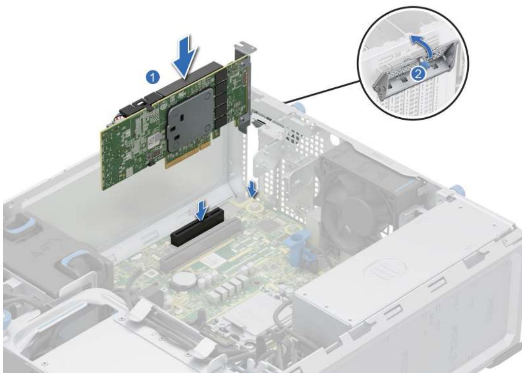
Ilustración 46. Instalación de una tarjeta de expansión
