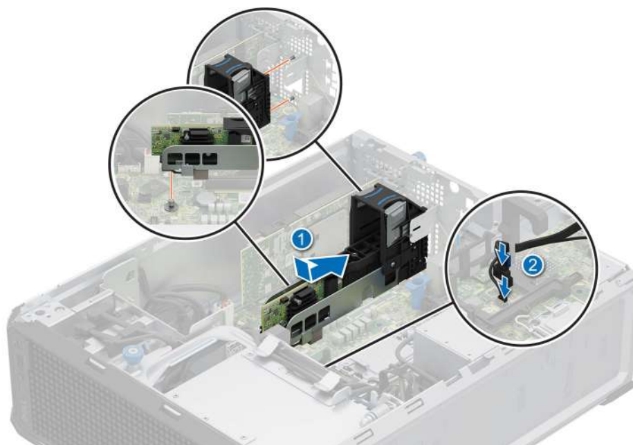
Ilustración 50. Instalación del módulo de BOSS-N1
