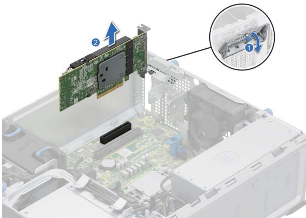
Ilustración 43. Extracción de una tarjeta de expansión
