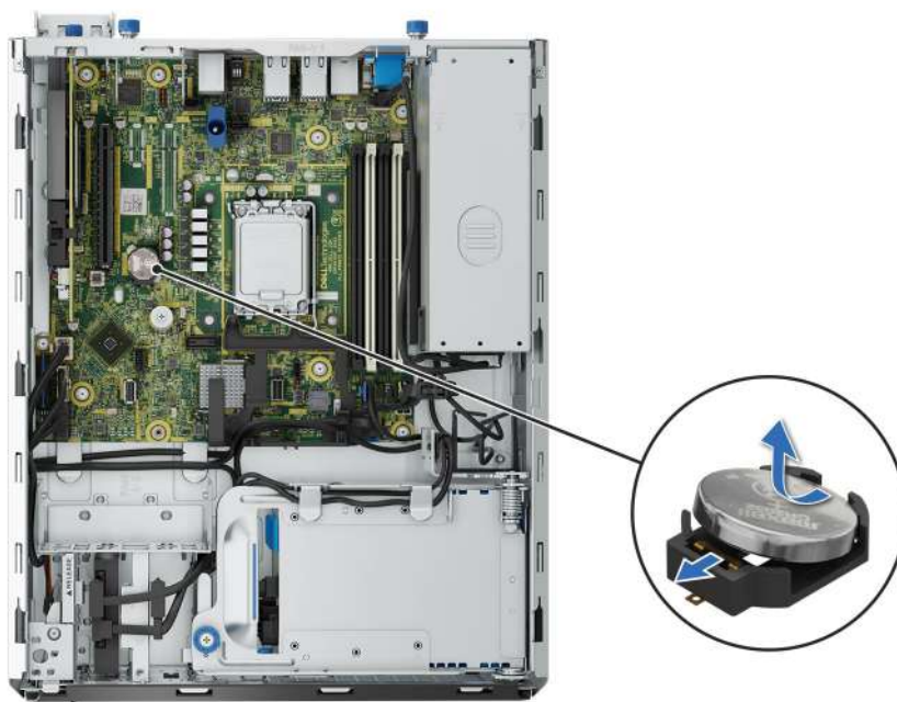
Ilustración 59. Extracción de la batería del sistema
