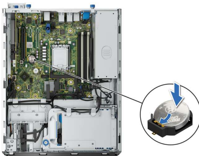
Ilustración 60. Instalación de la batería del sistema
