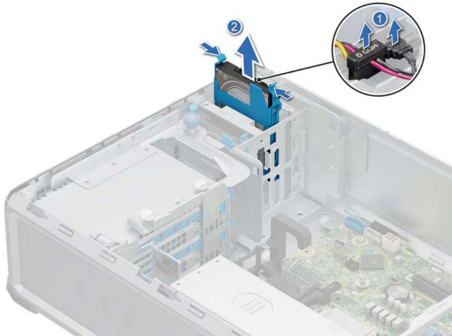
Ilustración 20. Extracción de la unidad de la caja de unidades
