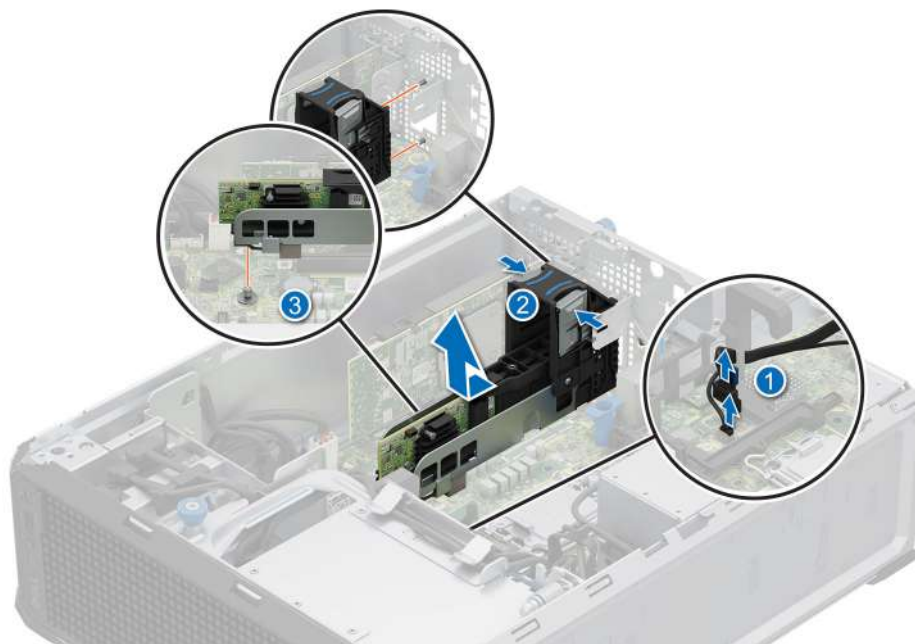
Ilustración 47. Extracción del módulo BOSS-N1
