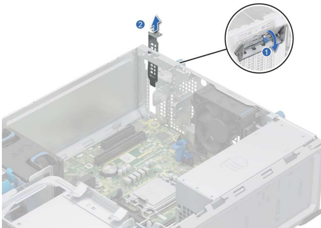
Ilustración 45. Extracción del soporte de relleno metálico
