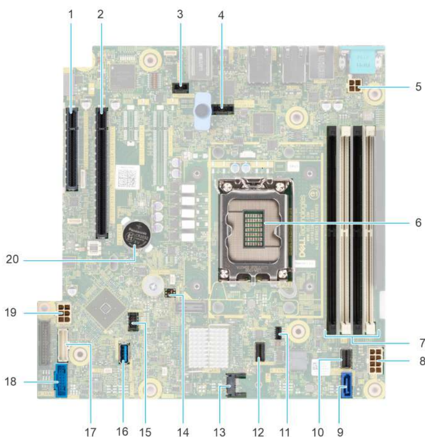
Ilustración 70. Diseño de la tarjeta madre
