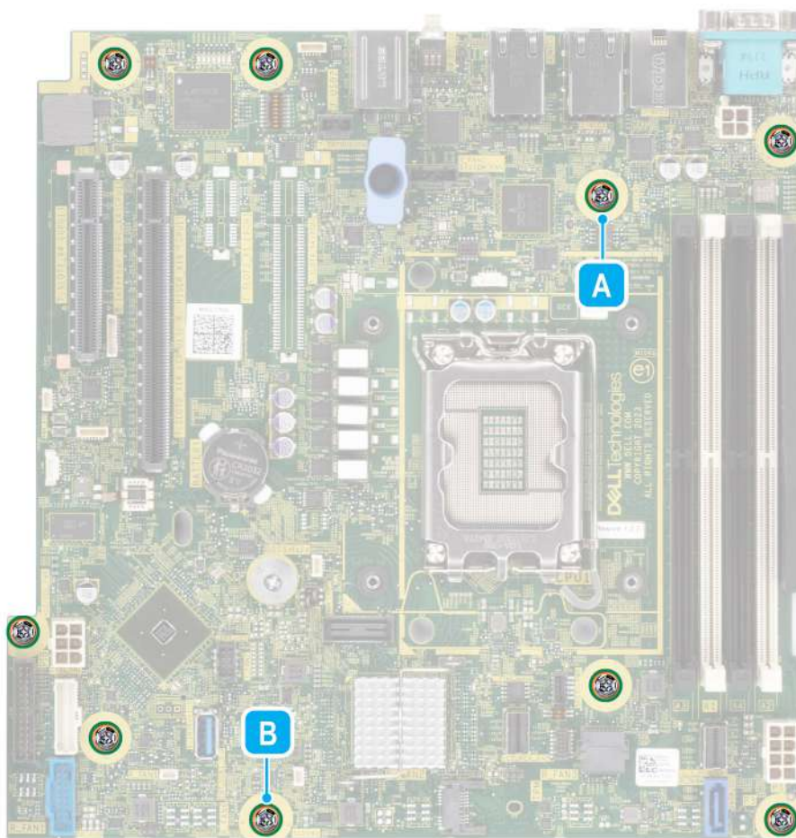
Ilustración 61. Ubicación del tornillo de la tarjeta madre
