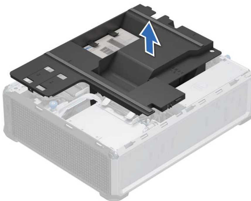
Ilustración 14. Extracción de la cubierta para flujo de aire
