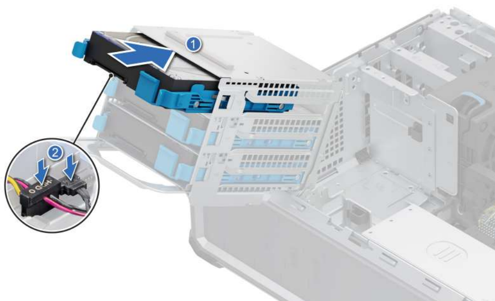
Ilustración 21. Instalación de un portaunidades
