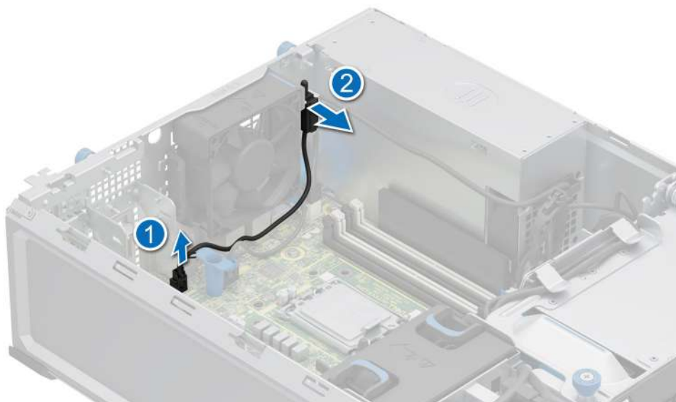
Ilustración 16. Extracción del módulo del switch de intrusión
