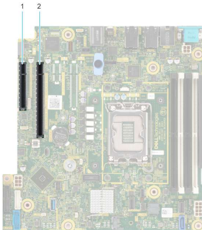
Ilustración 42. Ranuras del conector de PCIe en la tarjeta madre
