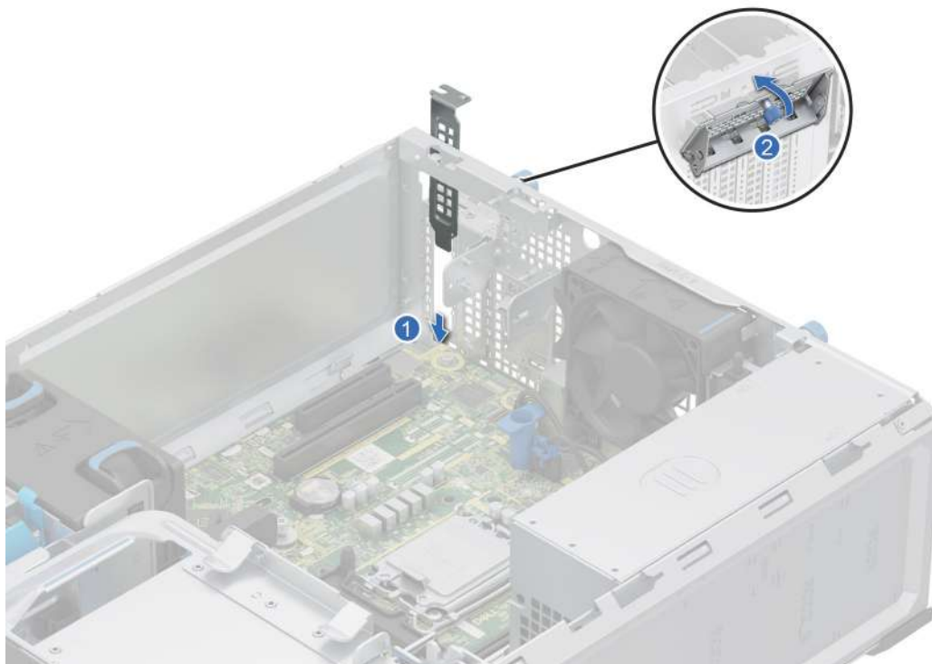
Ilustración 44. Instalación del soporte de relleno metálico
