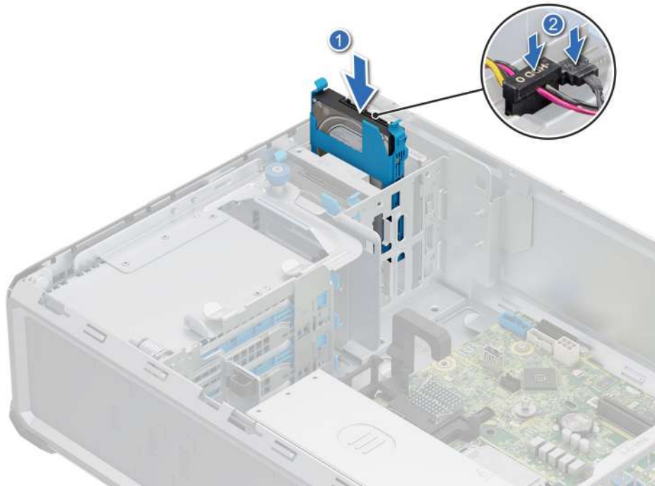
Ilustración 23. Instalación de un portaunidades
