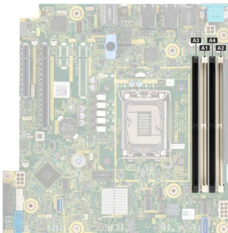
Ilustración 34. Ubicación de los conectores de memoria
