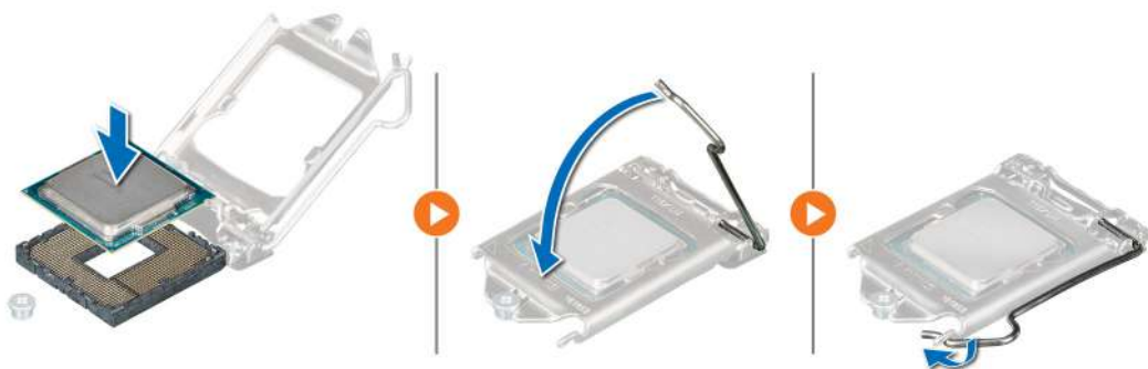
Ilustración 39. Instalación del procesador
