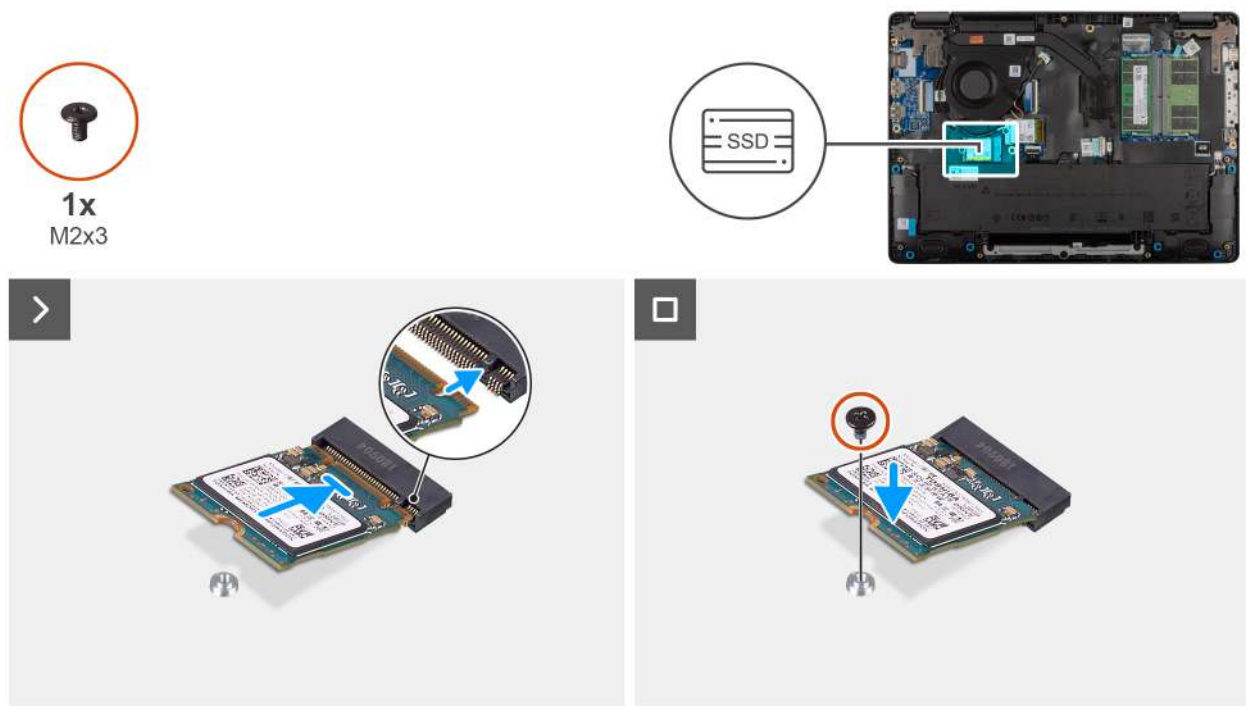
Ilustración 24. Instalación de SSD
