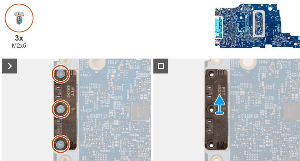
Ilustración 77. Extracción del módulo USB Type-C
