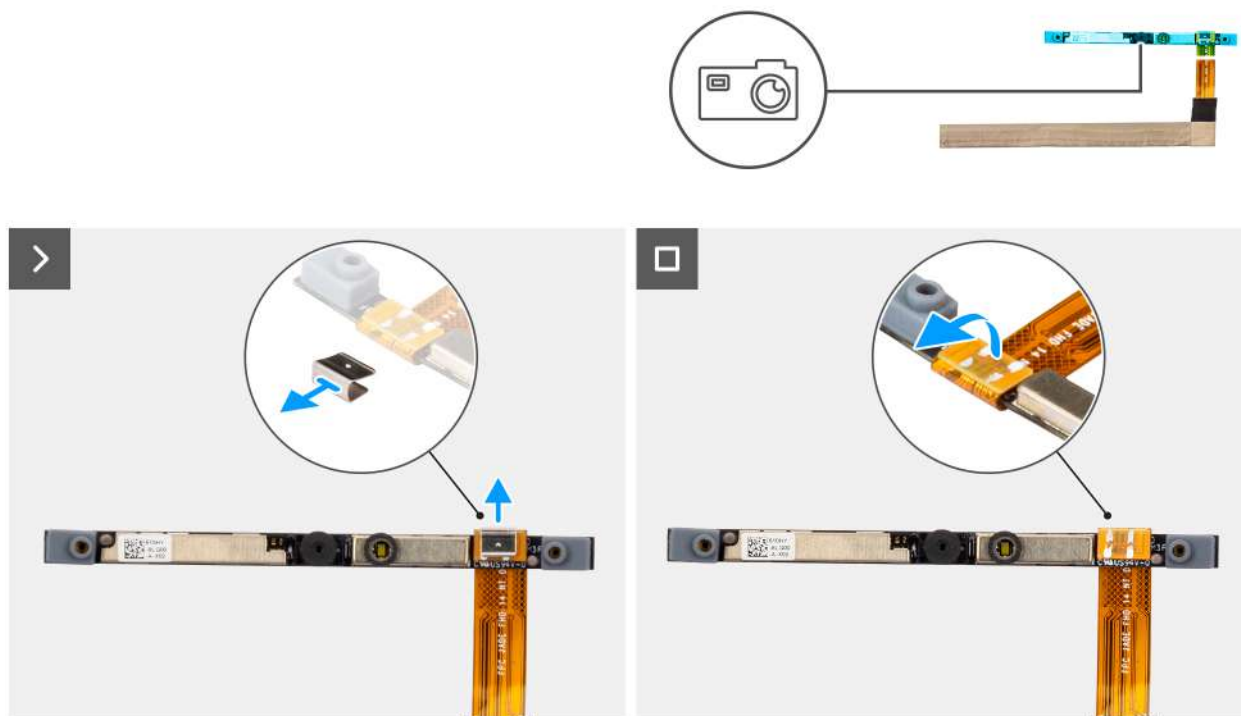
Ilustración 119. Extracción de la cámara
