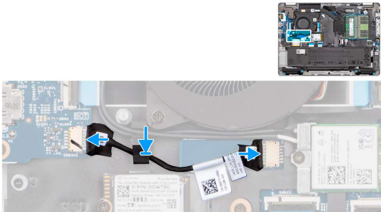
Ilustración 48. Instalación del cable de vPro
