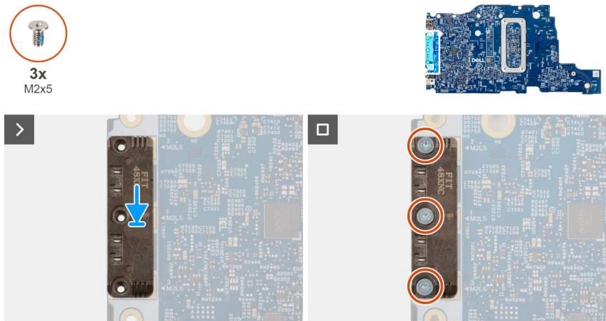
Ilustración 78. Instalación del módulo USB Type-C
