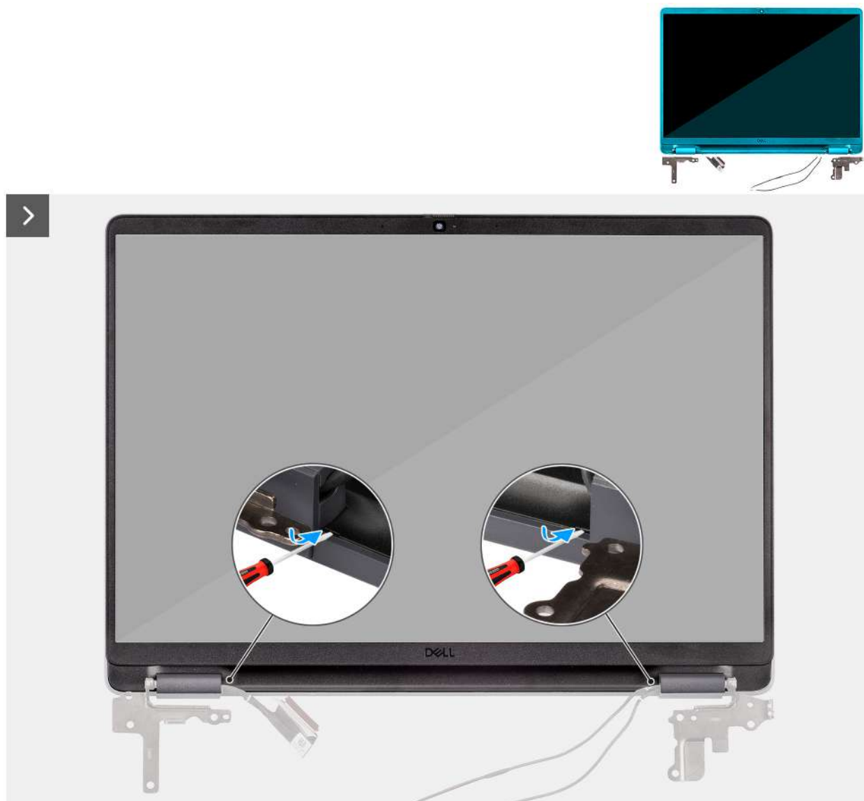
Ilustración 104. Extracción del embellecedor de la pantalla
