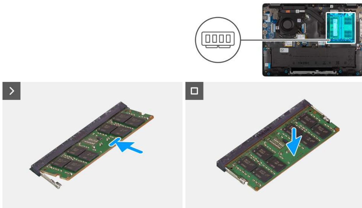
Ilustración 22. Instalación de los módulos de memoria
