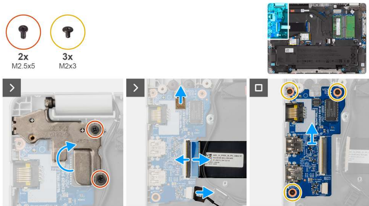
Ilustración 51. Extracción de la placa de I/O
