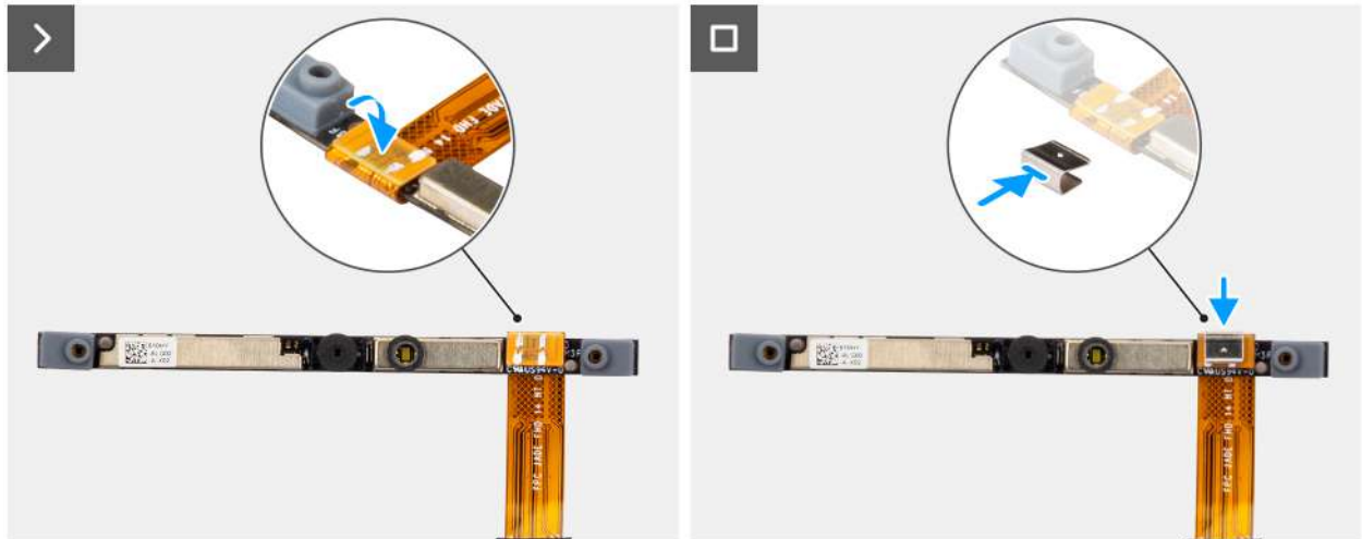
Ilustración 120. Instalación de la cámara
