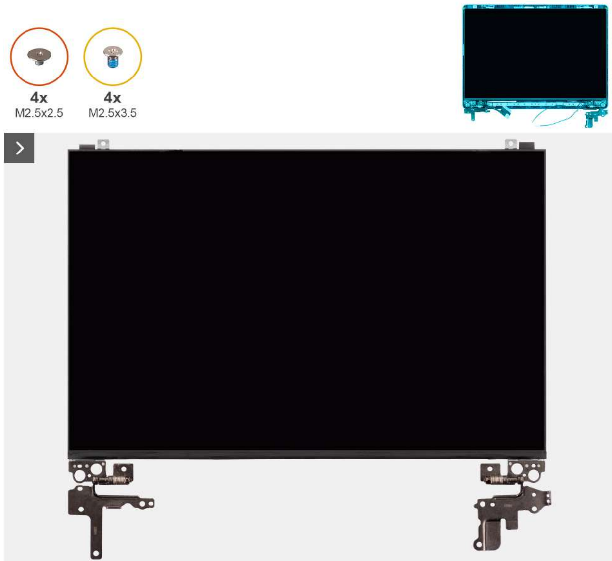
Ilustración 115. Instalación del ensamblaje del panel de pantalla
