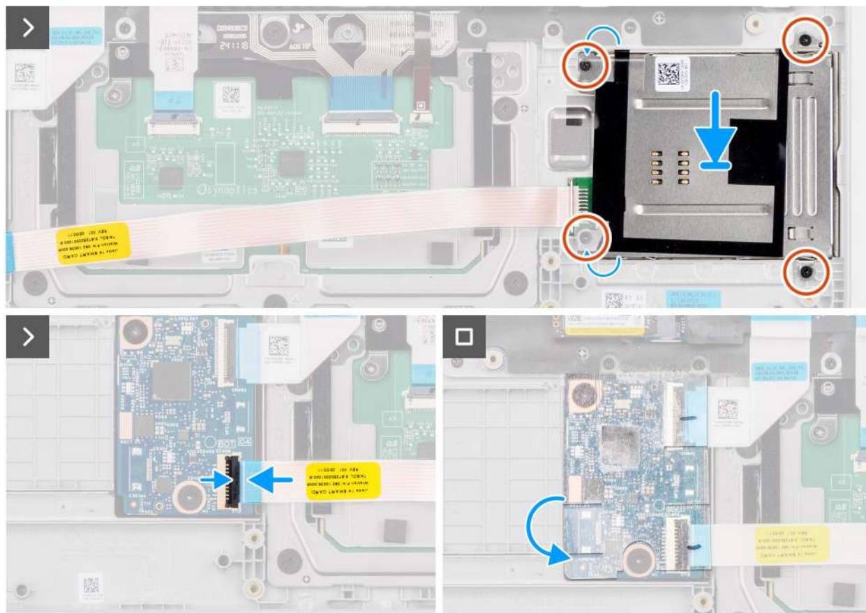
Ilustración 40. Instalación del lector de tarjetas inteligentes
