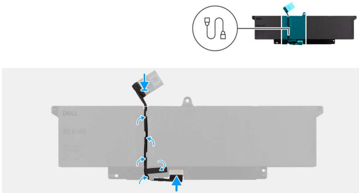
Ilustración 20. Instalación del cable de la batería
