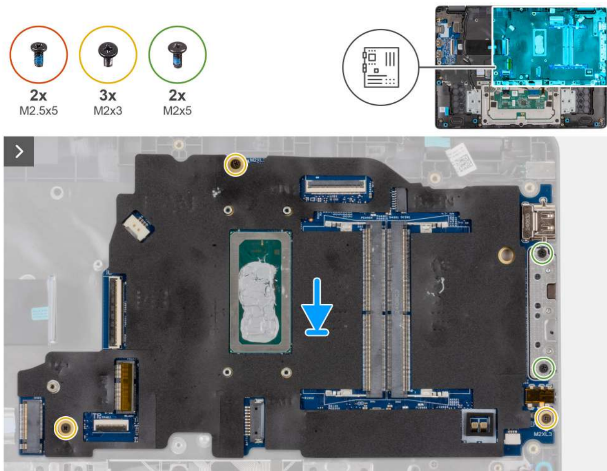
Ilustración 61. Instalación de la tarjeta madre
