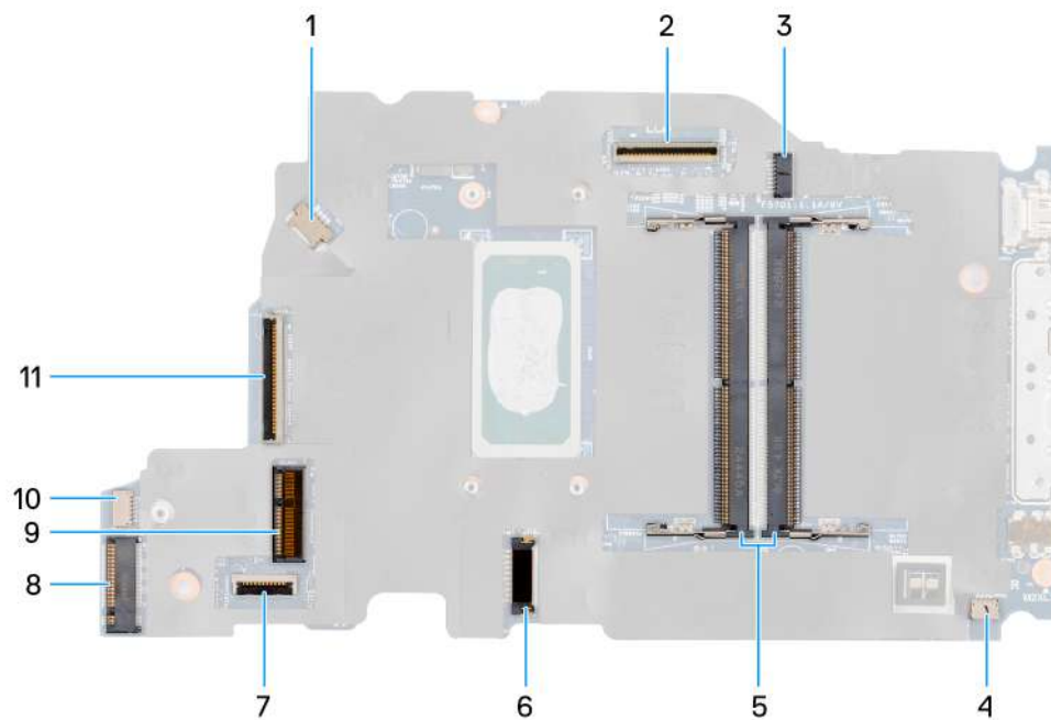
Ilustración 66. Conectores de la tarjeta madre
