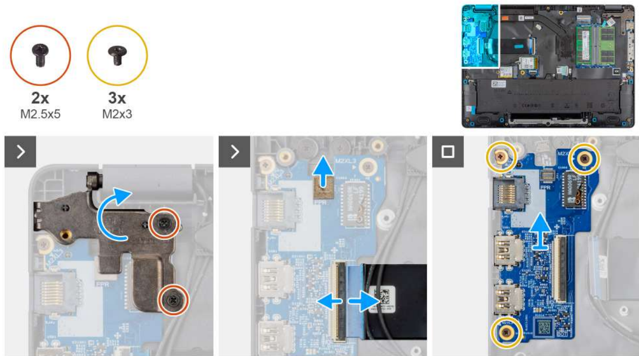
Ilustración 49. Extracción de la placa de I/O
