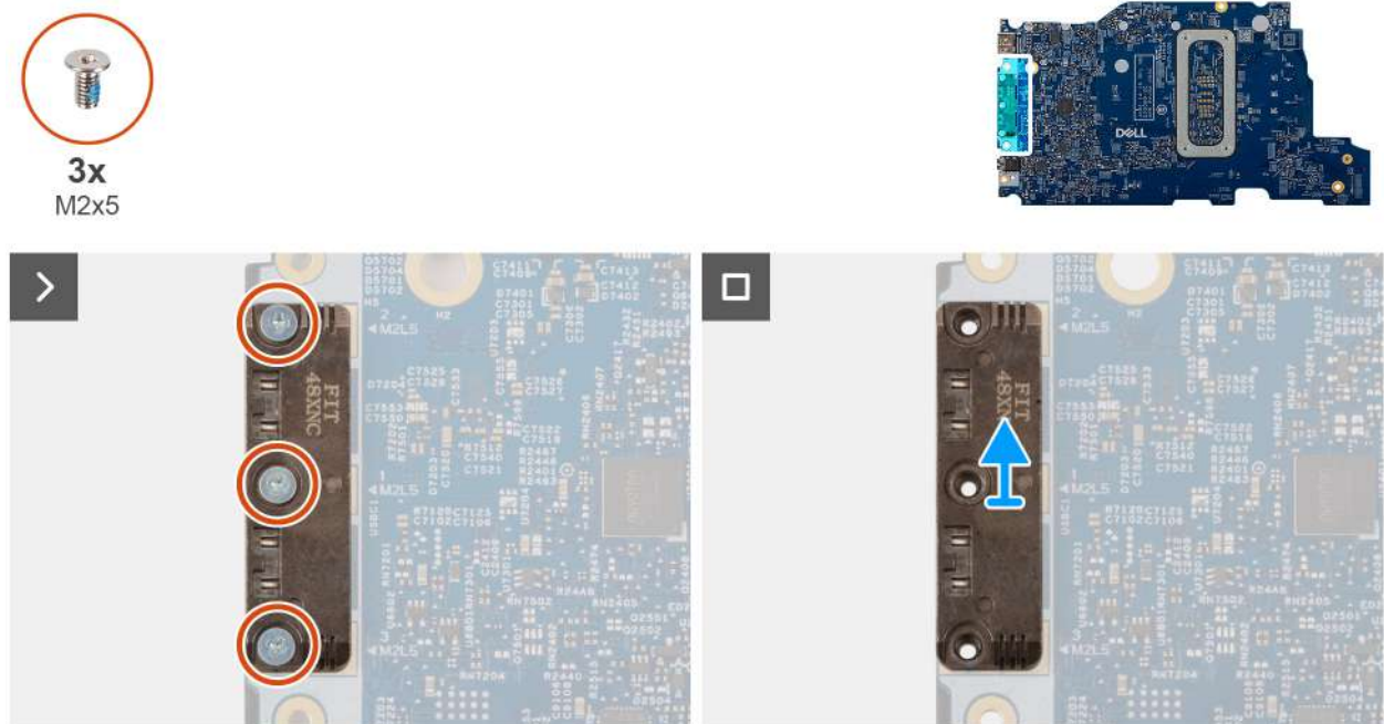
Ilustración 75. Extracción del módulo USB Type-C
